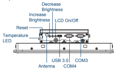
Left I/O
